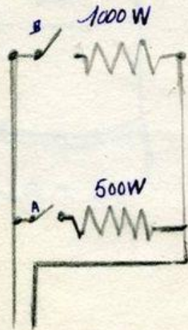
Radiateur à trois allures de chauffe
