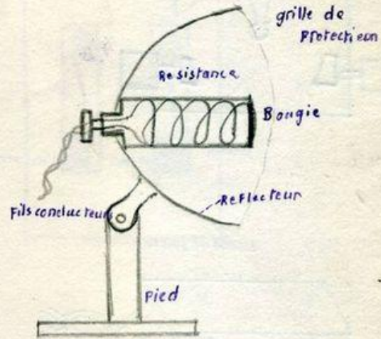
Radiateur à réflecteur
